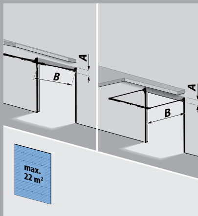
T 340 (B34), standard skinneresystem, bakopphengspakke + støtteprofil av stål
